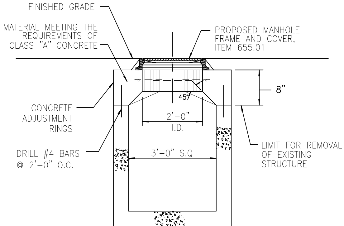
SECTION A-A
